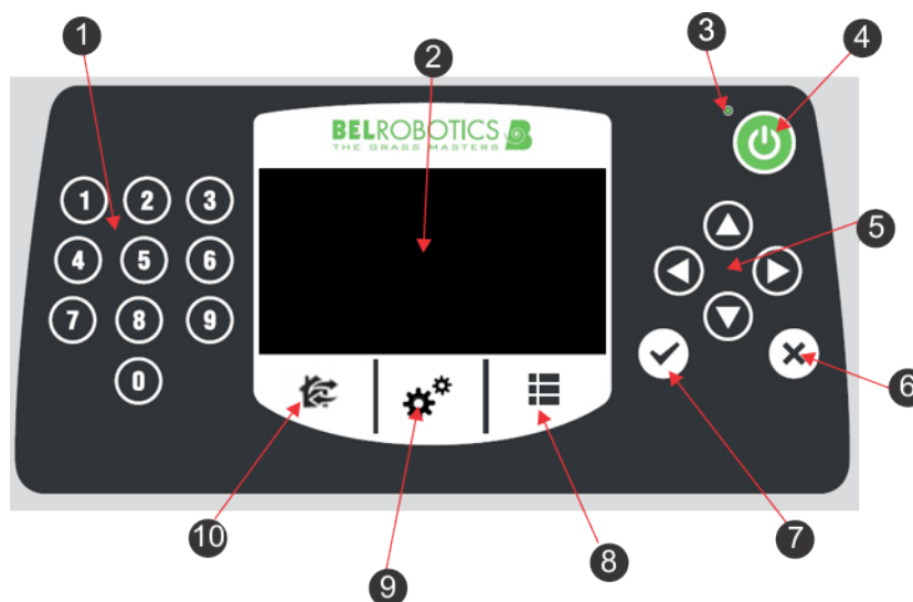
Afbeelding 18: Onderdelen van de gebruikersinterface
