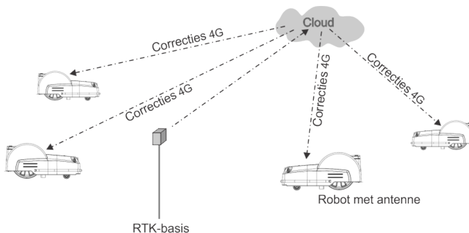
Afbeelding 23: Doorgeven van de correcties via 4G
