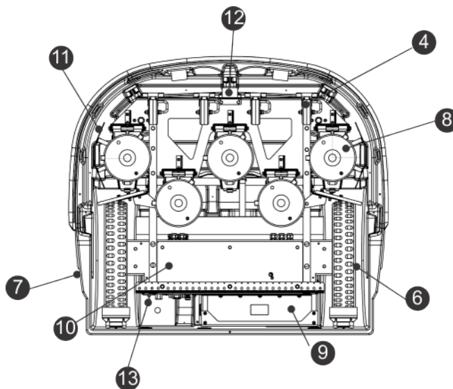
Afbeelding 4: Onderdelen aan de onderkant van de robot
